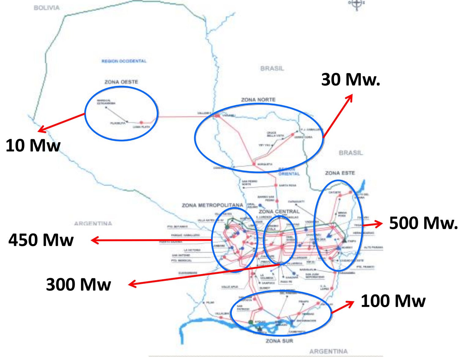
REPUBLICA DEL PARAGUAY - MAPA ELECTRICO AÑO 2014
